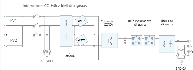
Schema elettrico
